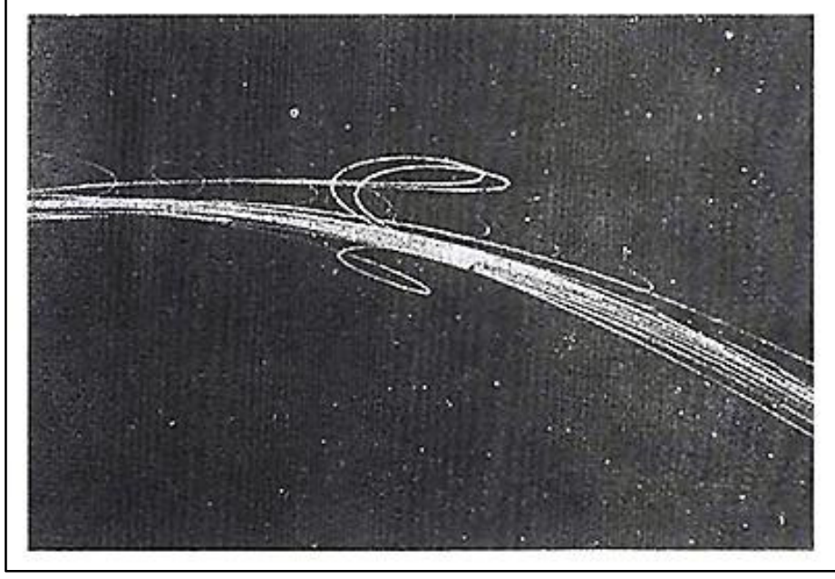
चित्र क्रमांक -1 : म्यूनख प्लॅनेटेरियम मध्ये ग्रहांच्या गतीची 17 वर्षांच्या कालखंडावर बतावणी करून घेण्यात आलेले छायाचित्र. काही ग्रह 'उलटे' जाताना दिसतात त्यांच्या मार्ग रेषांत फास तयार झालेले दिसतात. (म्यूनख प्लॅनेटेरियमच्या सौजन्याने)
